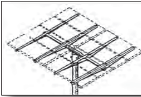
Montaje Cima-de-Poste
